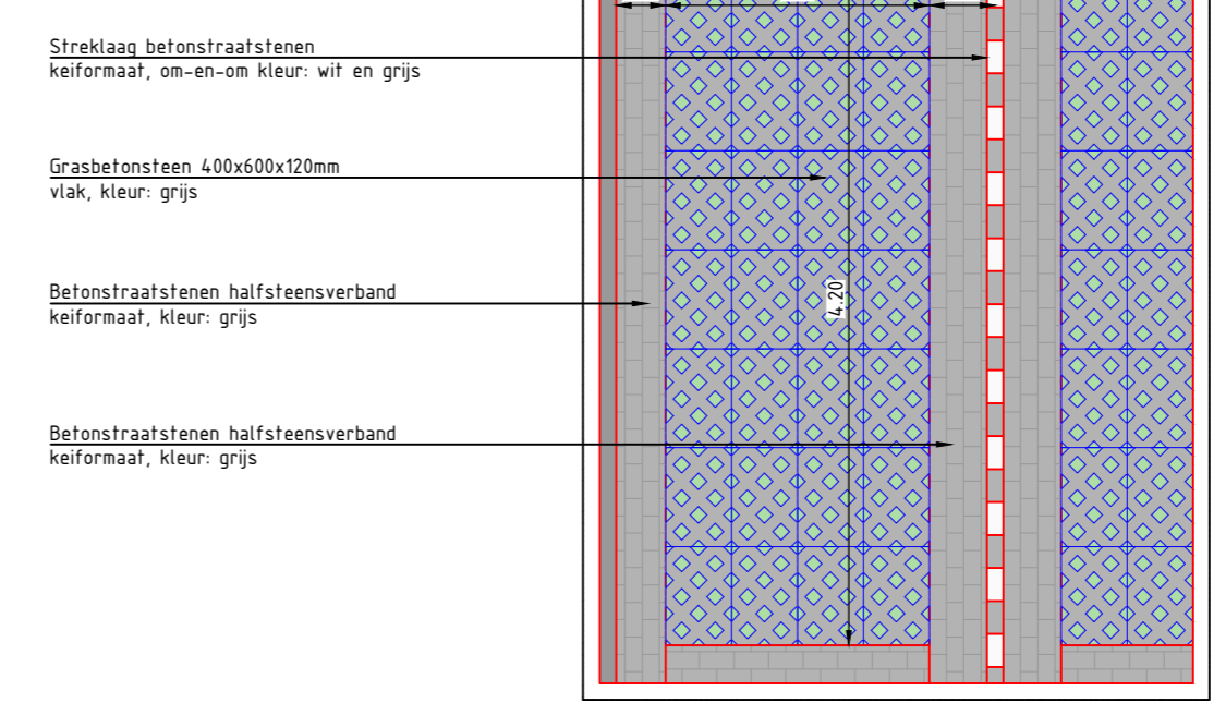
Detail 1: Principe parkeervakken van grasbetonstenen Schaal 1 : 50
